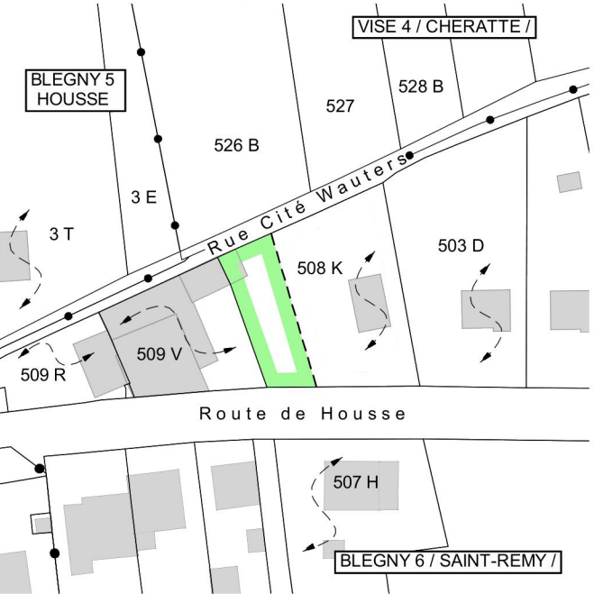
PLAN DE SITUATION ECH.: 1/1.000
